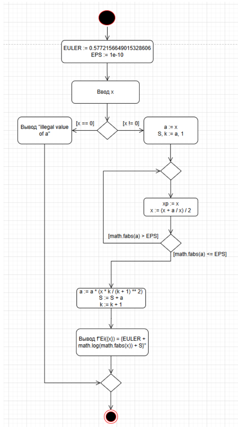
Рисунок 11. UML-диаграмма деятельности примера 5
